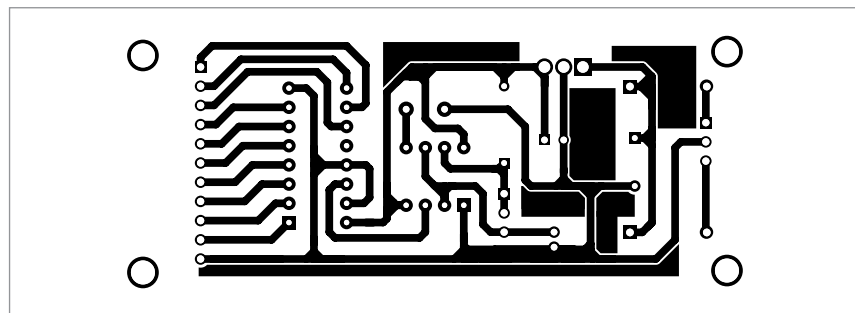
Fig. 3: Actual-size PCB layout
